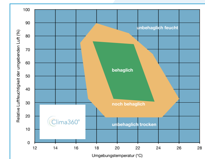
Behaglichkeitsdiagramm „Clima360“
