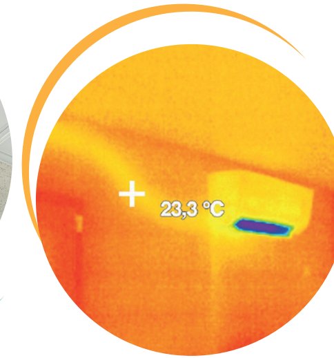
Thermografie Aufnahme einer Klimaanlage mit sichtbaren Unterputz Kältemittelleitungen
